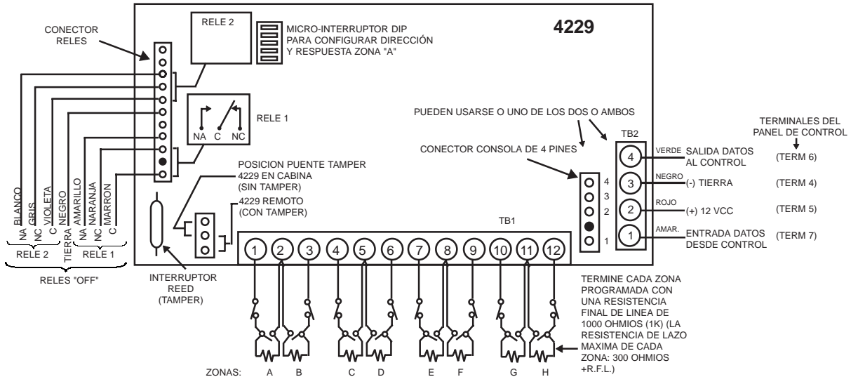
Figura 10. Cableado, 4219 y 4229 (Mostrado 4229)
